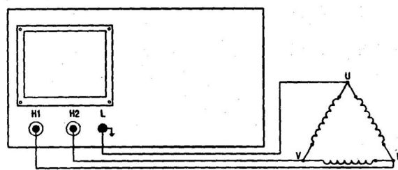
图 4-3 Δ（角）接法
